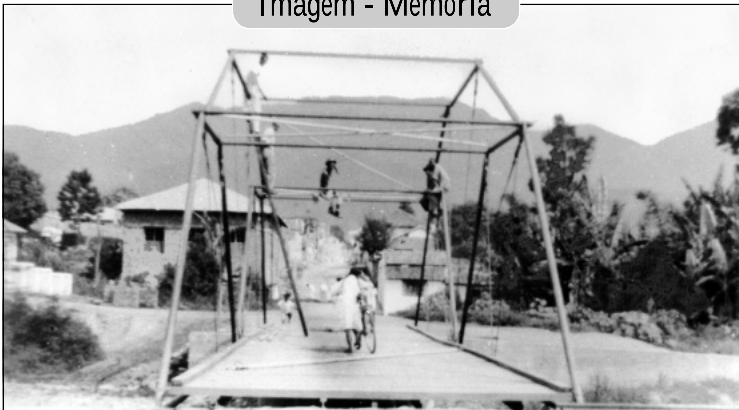
Projetada pelo Ten.Cel. José Pompeu Monte para ligar a Rua Major Carlos Ribeiro ao Largo da Estação “Rodrigues Alves”, esta ponte foi montada, anos mais tarde, em dois outros locais da cidade, até ser definitivamente retirada em 1990. Na foto, montagem da “Ponte dos Ex-Alunos”, como ficou conhecida, à Rua Cel. Pederneiras, no início da década de 50 do século 20.
