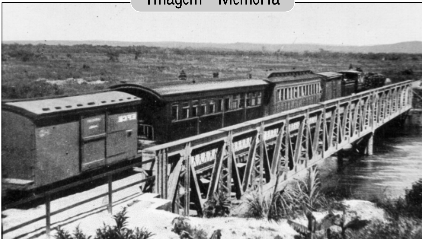
Comboio proveniente de Piquete transpondo a ponte metálica sobre o rio Paraíba do Sul, em Lorena: trecho do ramal-férreo Lorena-Benfica.
